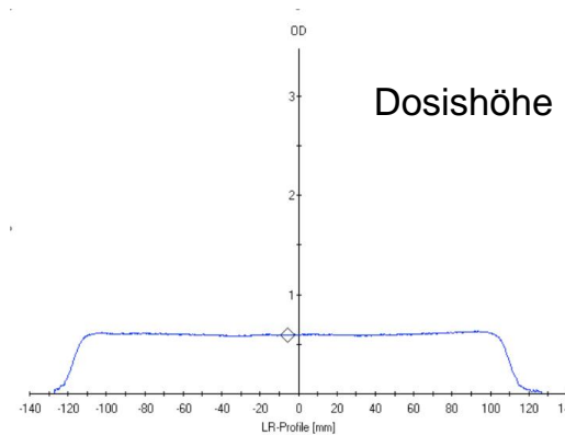
Resultierende gleichmäßige Dosis vermessen
